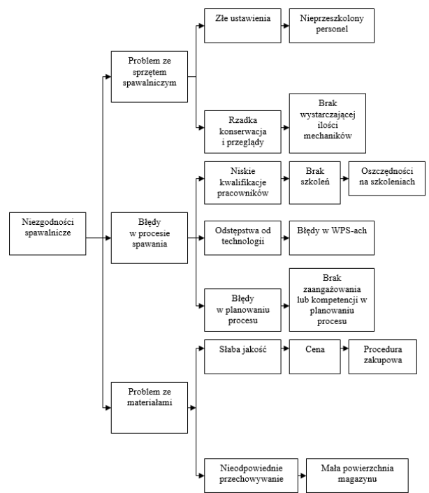
Rys. 6. Diagram WHY-WHY dla analizy przyczyn niezgodności spawalniczych
